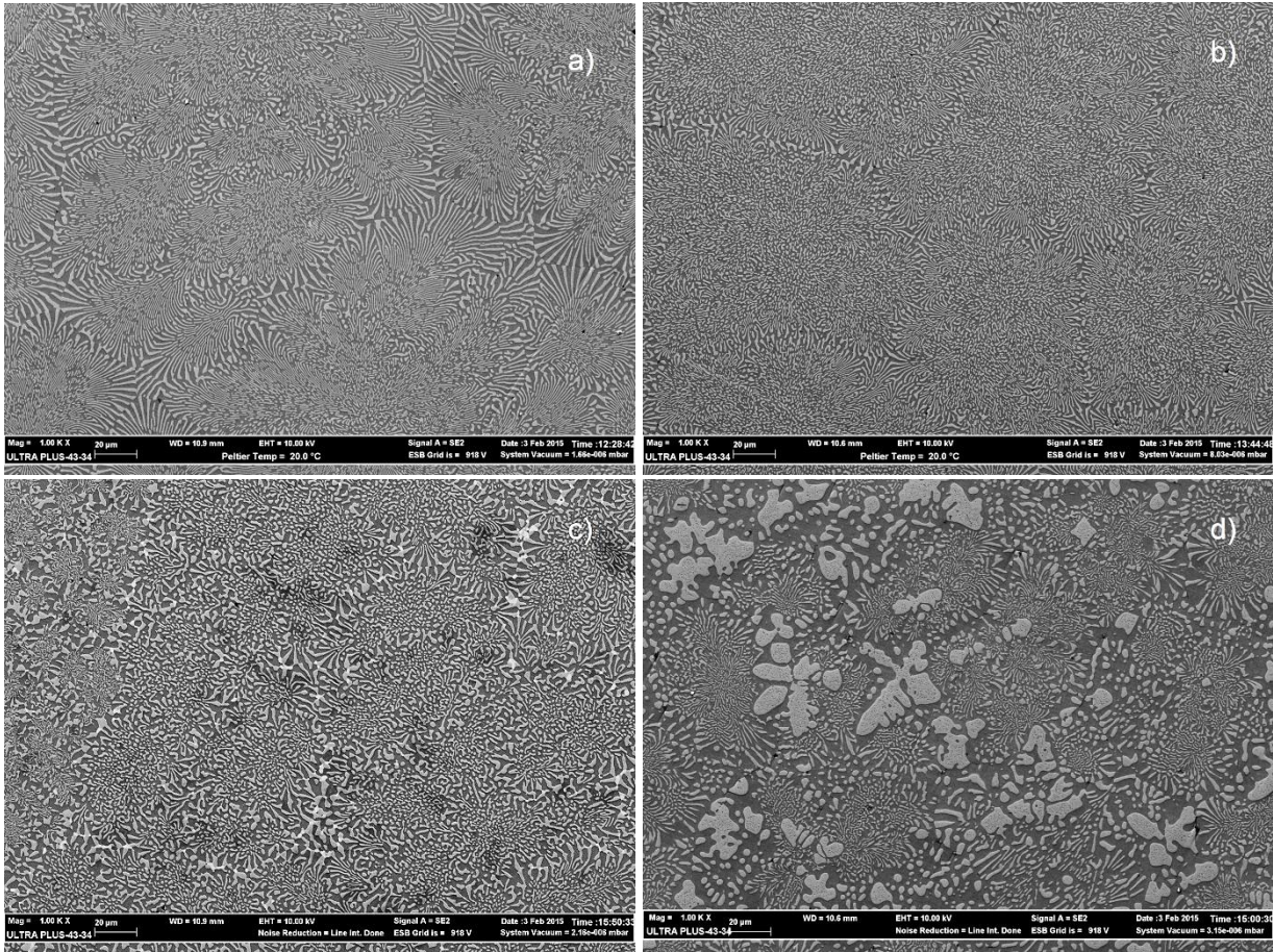
Fig. 1 The microstructure of alloys; a) NiAl-Cr(Mo) b) NiAl-Cr(Mo)-0.1Fe c) NiAl-Cr(Mo)-1Nb and d) NiAl-Cr(Mo)-4Ti.
